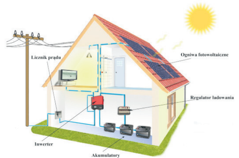
Schemat instalacji fotowoltaicznej
