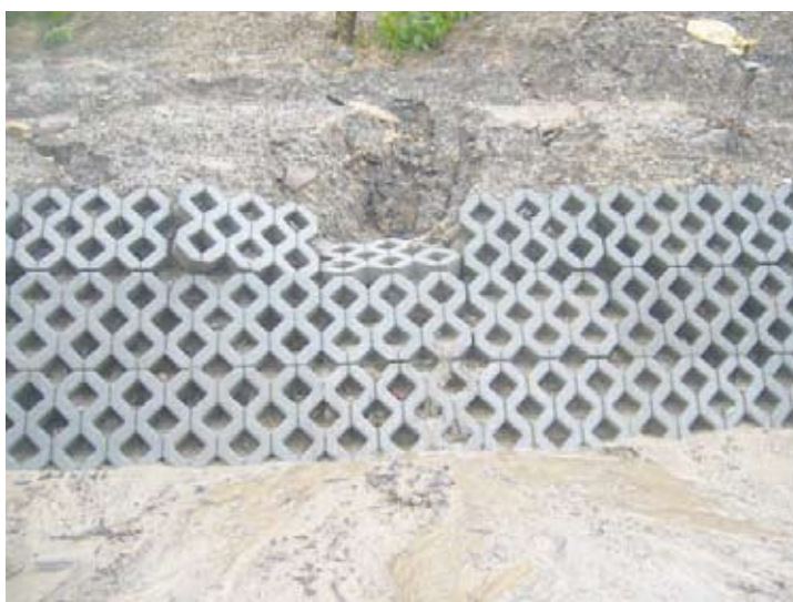
Pod wpływem deszczu osuwająca się ziemia poprzewracała płytki. Foto: Dariusz Nowak
